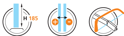
Binario di scorrimento «colibrì»
